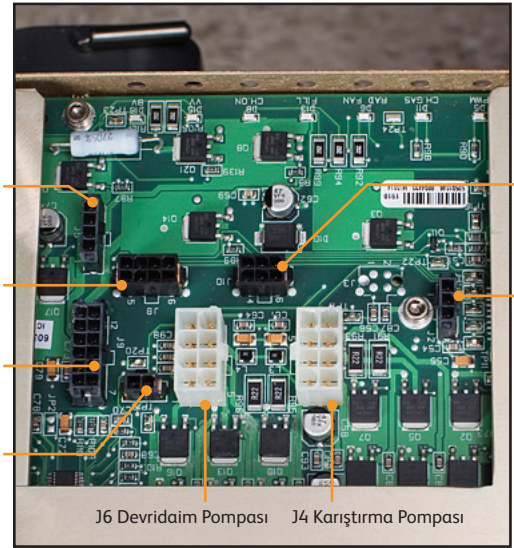
Şek. 8-15 I/O Devre Kartı bağlantıları
