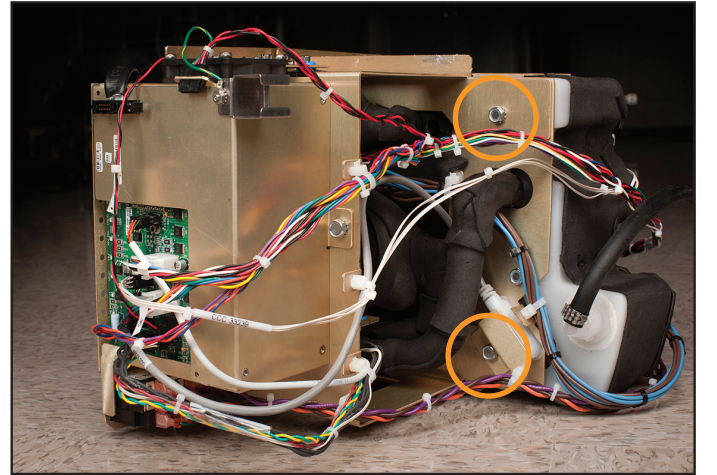
Şek. 8-25 Dahili bileşenler (arkadan görünüm); daireler, çıkarılacak cıvataları gösterir (Adım 1)
