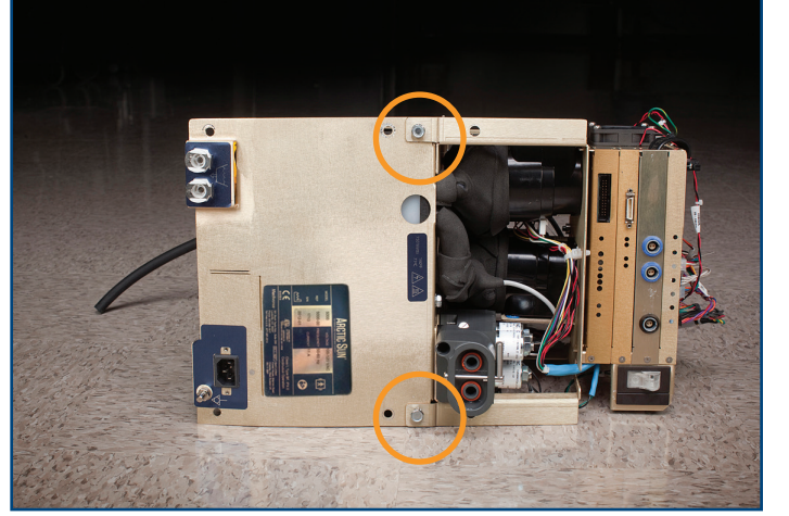
Şek. 8-24 İki bölüme ayrılmadan önce dahili bileşenler (önden görünüm)
