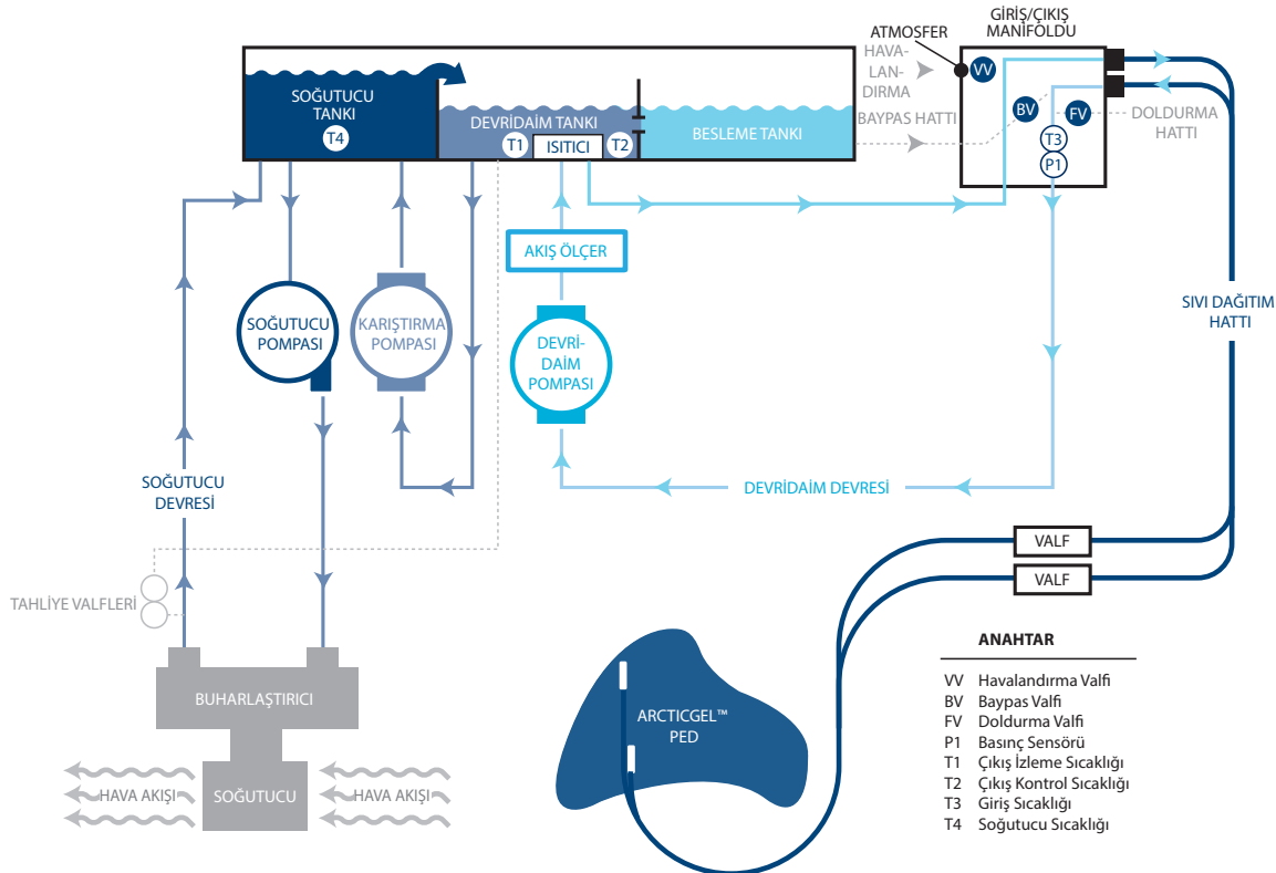
Şek. 2-1 Hidrolik Şeması
