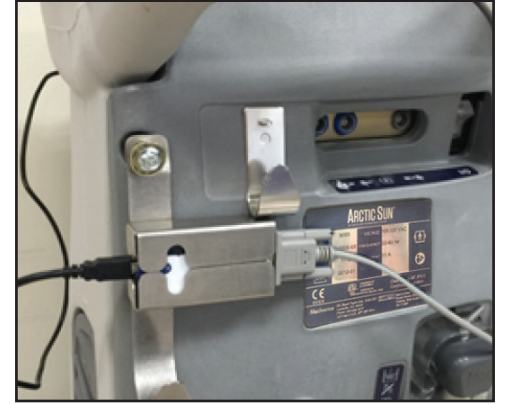
Şek. 8-74 TIM'i yerleştirin ve kabloları bağlayın (Adım 3-5)
