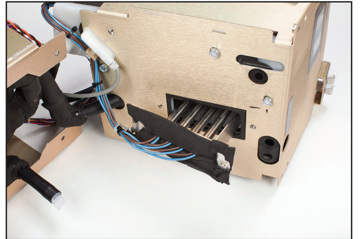
Şek. 8-50 Isıtıcıyı çıkarın (Adım 4)
