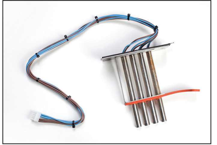
Şek. 8-48 Isıtıcı
