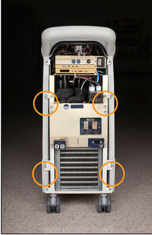
Şek. 8-11 4 cıvatayı çıkarın (Adım 1)
