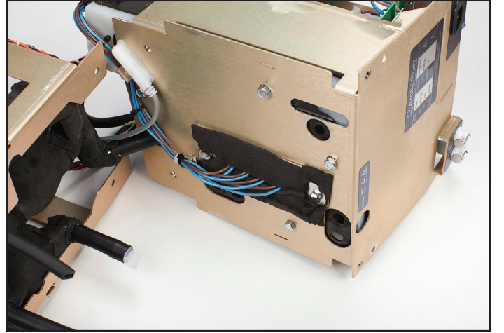
Şek. 8-49 Çıkarılacak kablo bağlarının gösterildiği Tank ve Isıtıcı (Adım 2)
