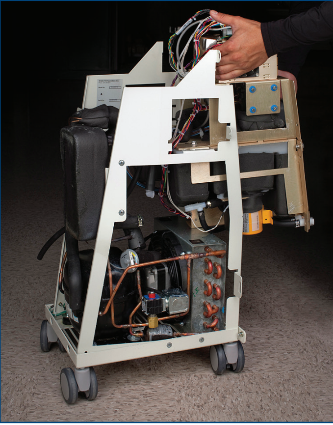
Şek. 8-23 Dahili bileşenleri kaldırarak çıkarın (Adım 4)
