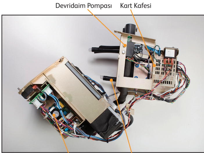
Şek. 8-26 İki bölüme ayrılan dahili bileşenler (2 görünüm)
