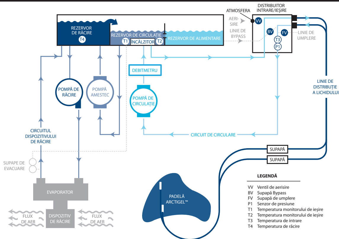
Fig. 2-1 Schema hidraulică
