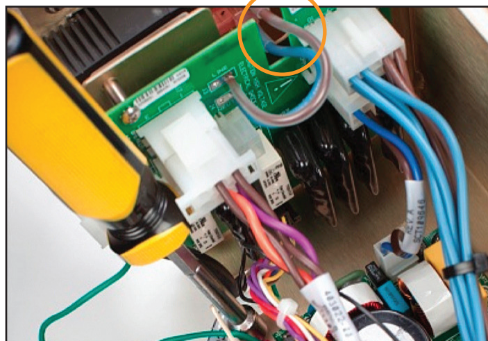
Fig. 8-69 Card de circuit de tensiune de rețea în poziție, cu conexiunile în poziție
