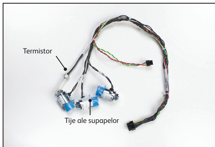
Fig. 8-59 Cablajul distribuitorului (prezentat cu capace de protecție)
