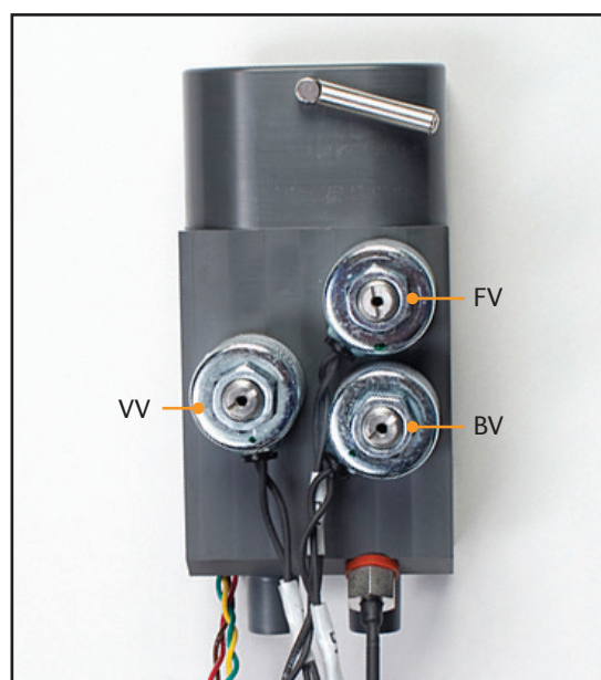
Fig. 8-62 Distribuitorul, cu indicarea pozițiilor celor 3 solenoizi (pasul 8)
