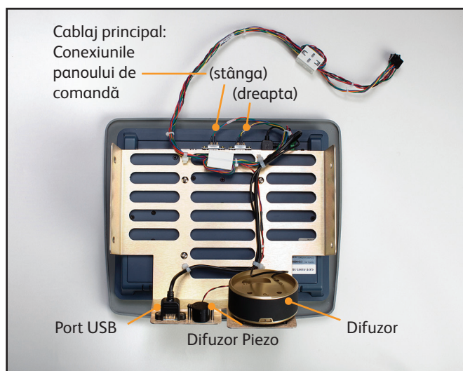
Fig. 8-55 Panou de comandă (vedere din spate)
