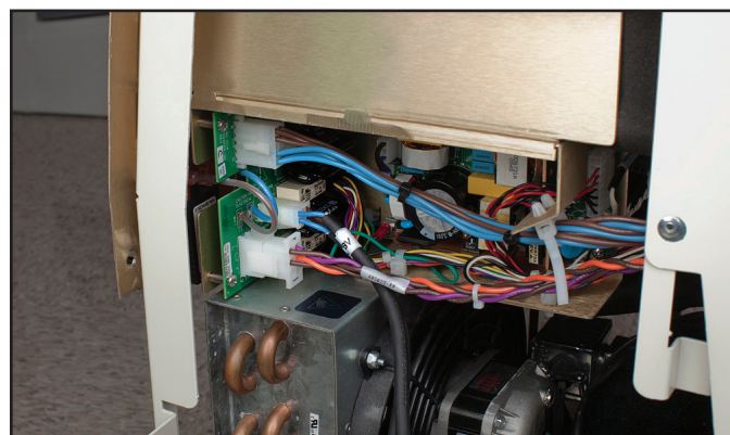
Fig. 8-20 Deconectați cablul gri al conexiunii de alimentare a dispozitivului de răcire; locația indicată (pasul 2)
