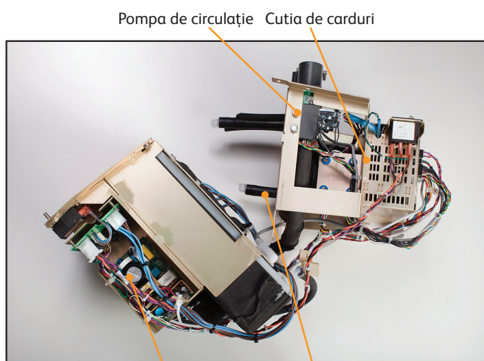
Fig. 8-26 Componente interne separate în două secțiuni (2 vederi)
