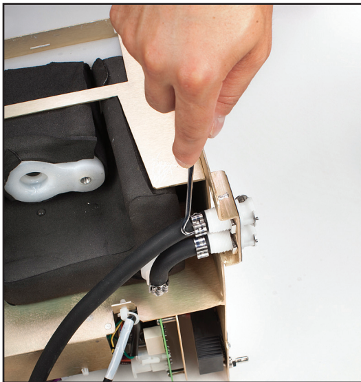
Fig. 8-43 Åpne klemmen som forbinder kjølerpumpeslangen til dreneringsventilen
