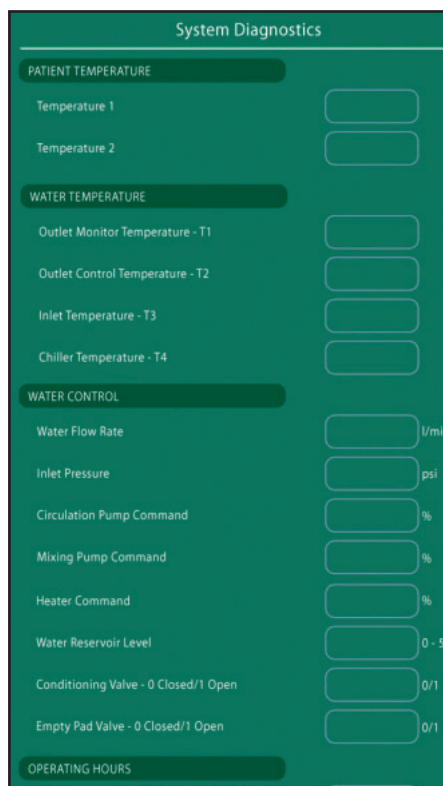
Fig. 7-1 Systemdiagnostikk
