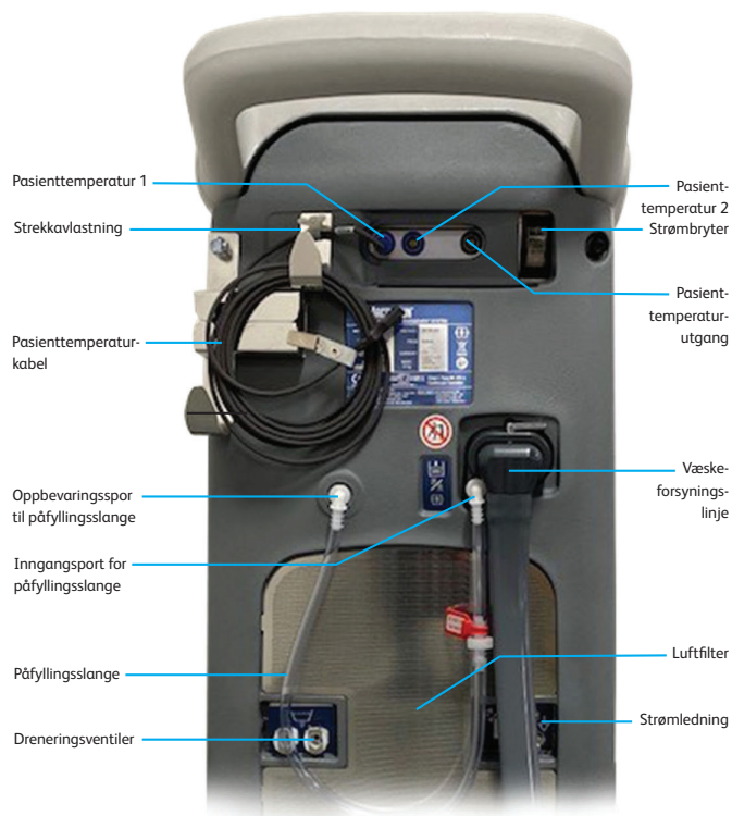
Fig. 1-1 ARCTIC SUN™-temperaturstyringssystemets kontrollmodul
