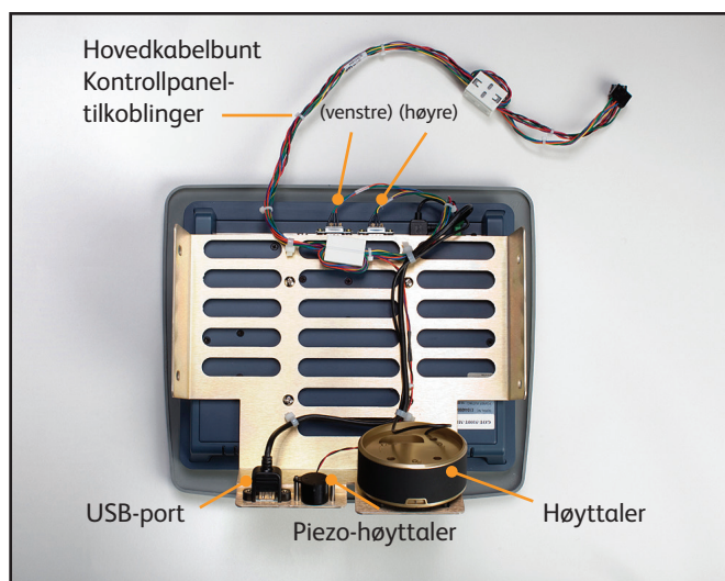
Fig. 8-55 Kontrollpanel (sett bakfra)
