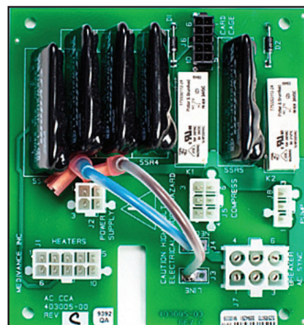
Fig. 8-7 Nätpänningens kretskort
