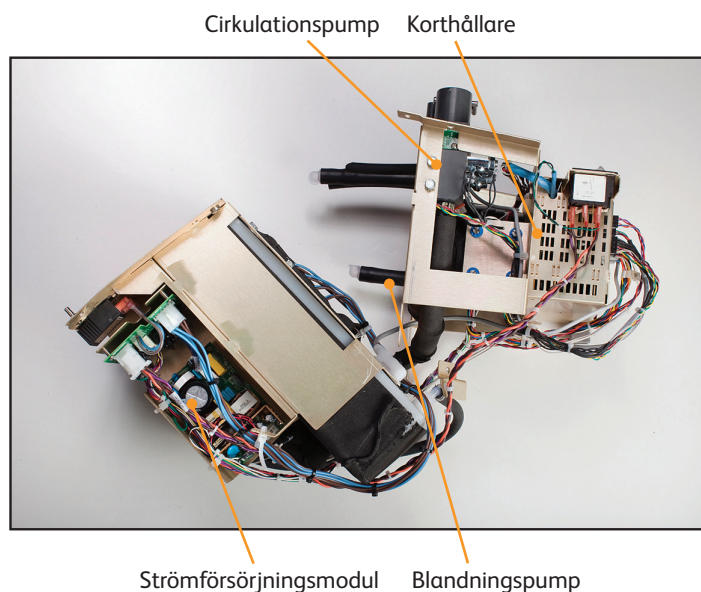
Fig. 8-26 Interna komponenter uppdelade i två delar (2 vyer)
