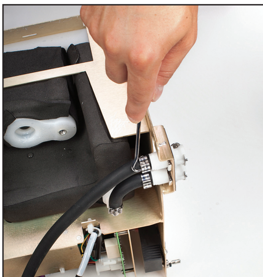
Fig. 8-43 Öppna klämman som ansluter kylarpumpslangen till tömningsventilen
