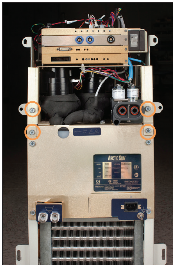
Fig. 8-16 Ta bort fyra bultar (steg 1)
