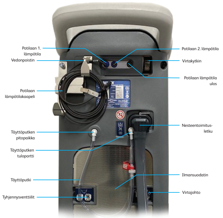
Kuva 1-1 ARCTIC SUN™ -lämpötilanhallintajärjestelmän kontrollointimoduuli
