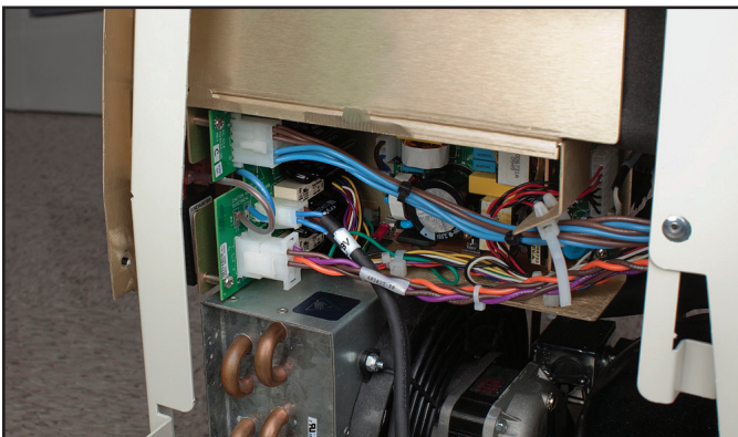
Kuva 8-20 Irrota jäädyttimen virtaliitännän harmaa kaapeli; sijainti ilmoitettu (vaihe 2)
