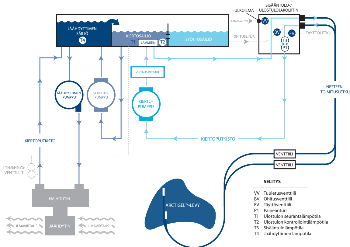
Kuva 2-1 Hydraulinen kaavio
