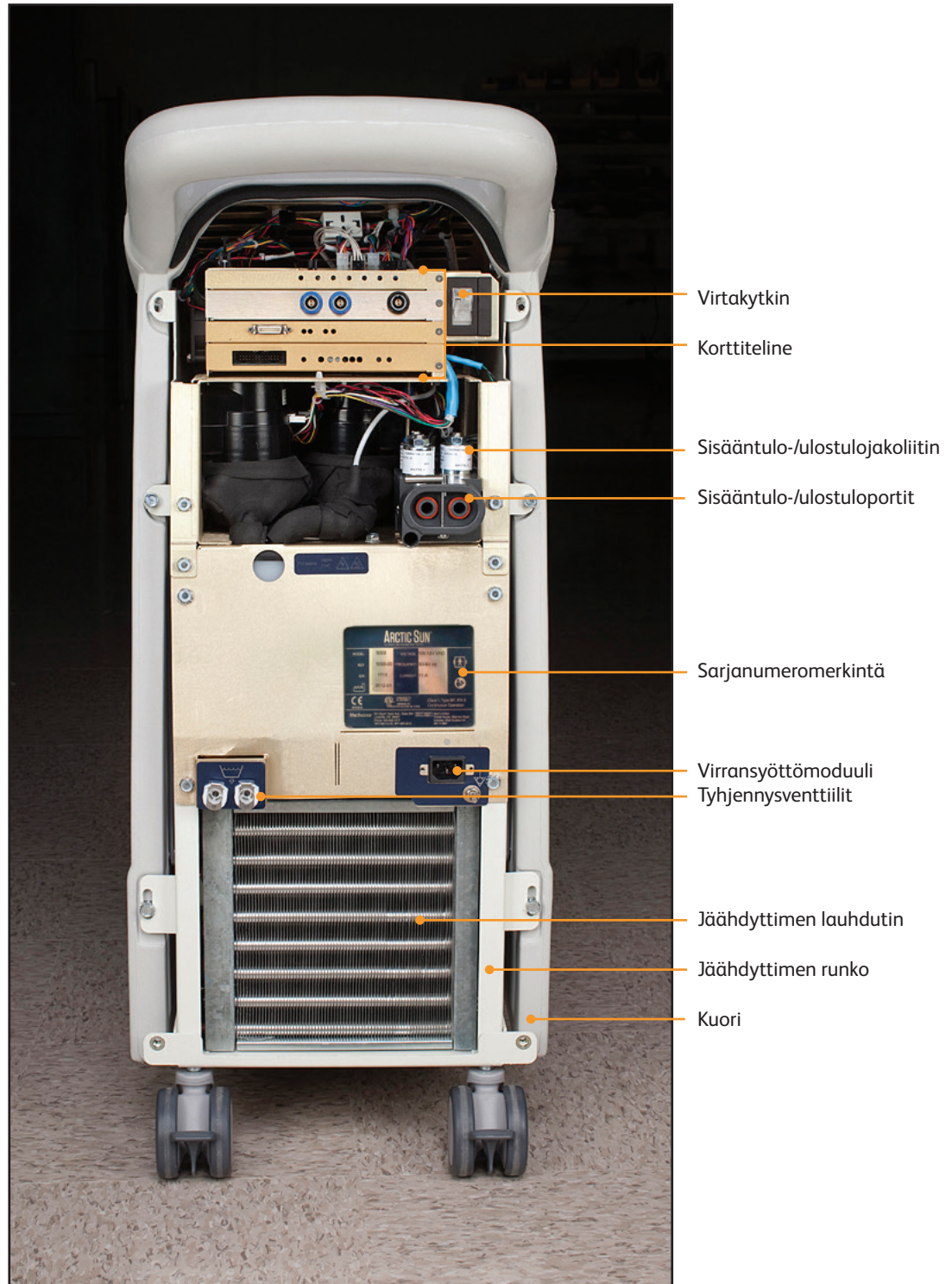
Kuva 8-1 Kontrollointimoduuli, näkymä takaa takapaneelin poistamisen jälkeen
