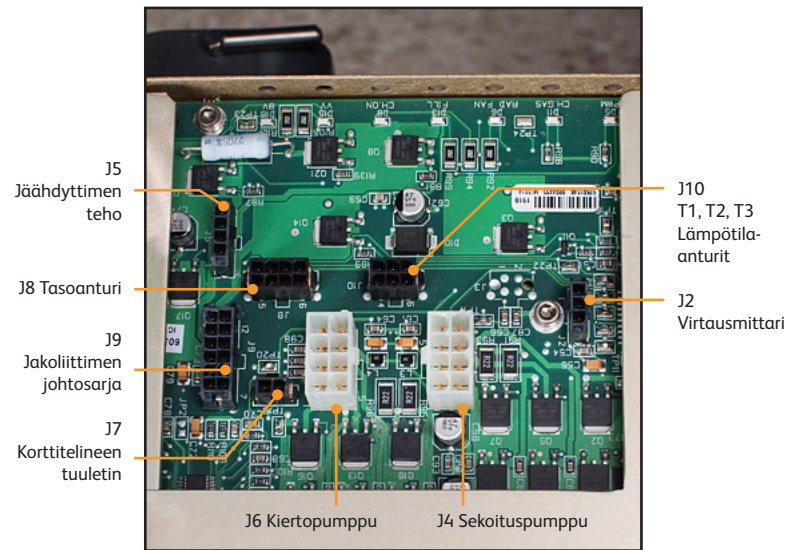
Kuva 8-15 I/O-piirikorttiliitännät
