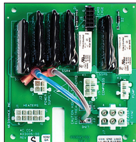
Kuva 8-7 Verkköjännitepiirikortti
