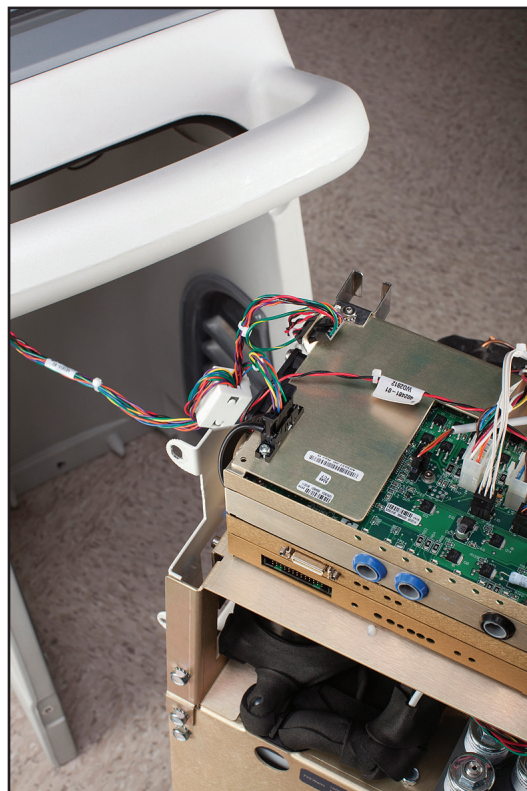
Kuva 8-12 Poistettavat kaapelisarjat (vaihe 3)
