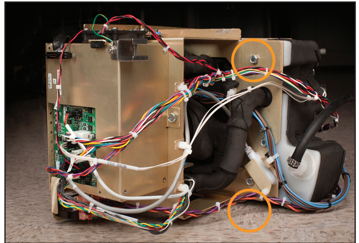
Kuva 8-25 Sisäkomponentit (näkömä takaa); ympyrät ilmaisevat irrotettavat pultit (vaihe 1)
