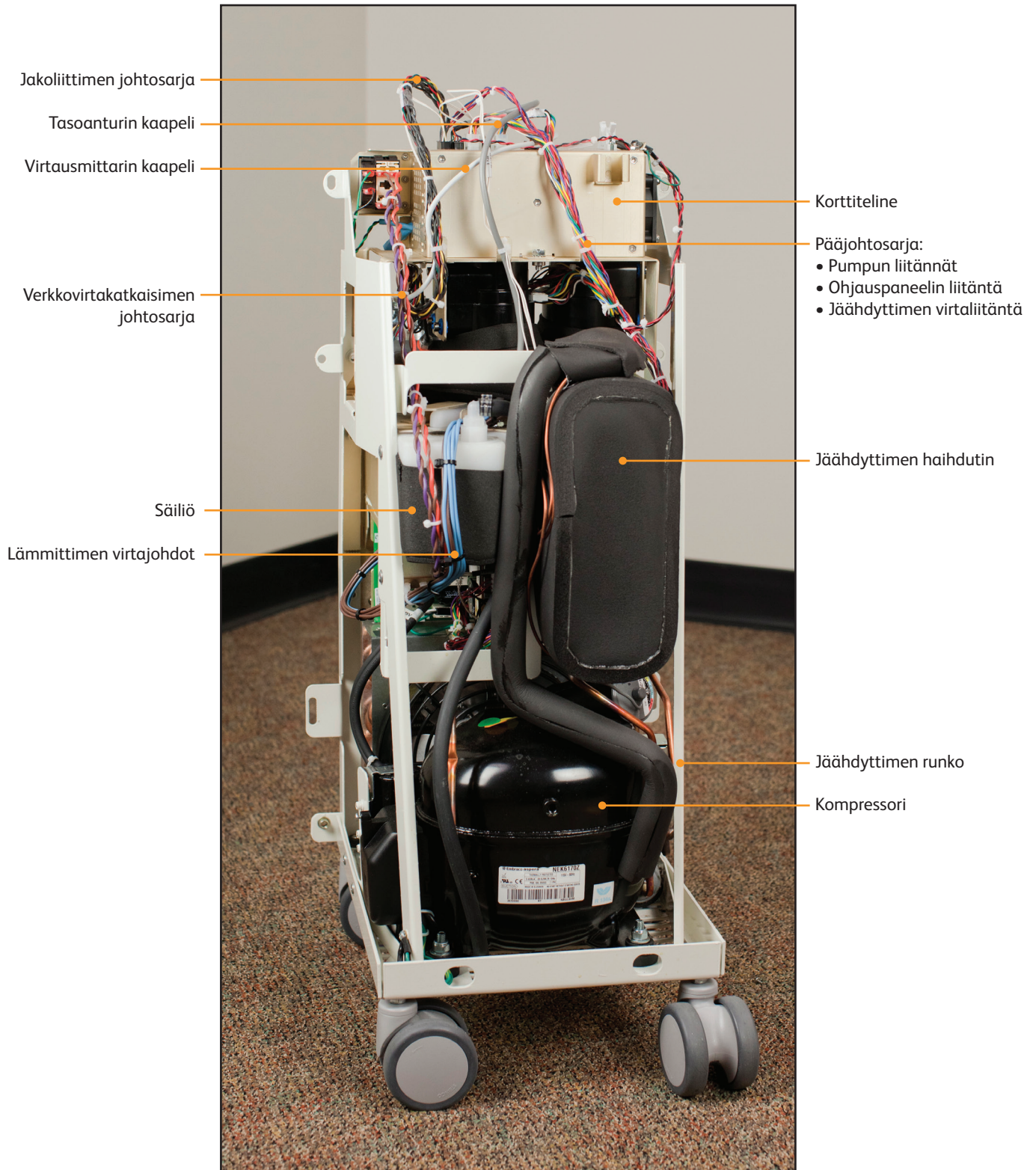
Kuva 8-2 Kontrollointimoduuli, näkymä sisältä etupuoelta
