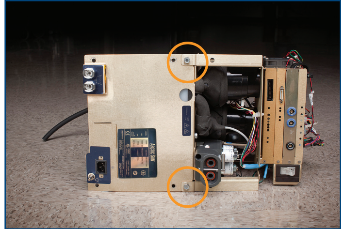
Kuva 8-24 Sisäkomponentit ennen niiden erottamista kahteen osaan (näkömä edestä)
