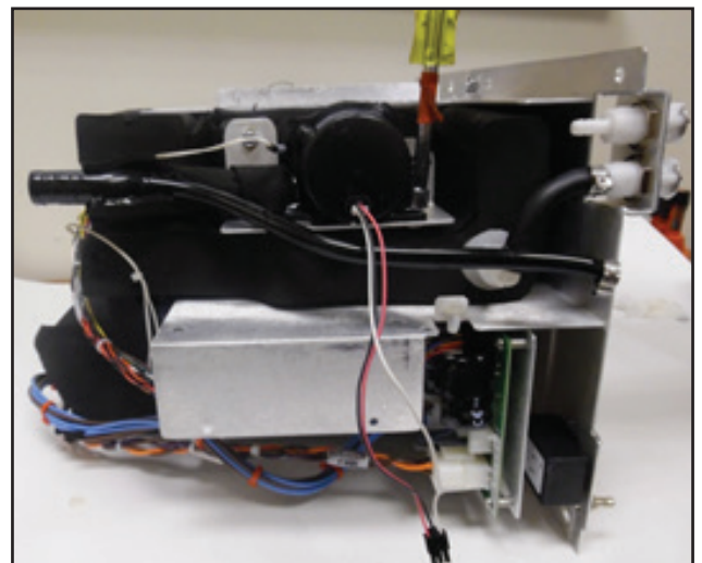
Fig. 8-46 Retire los pernos (paso 4)
