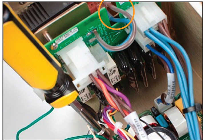
Fig. 8-69 Tarjeta del circuito de tensión principal en su posición, con las conexiones en su lugar
