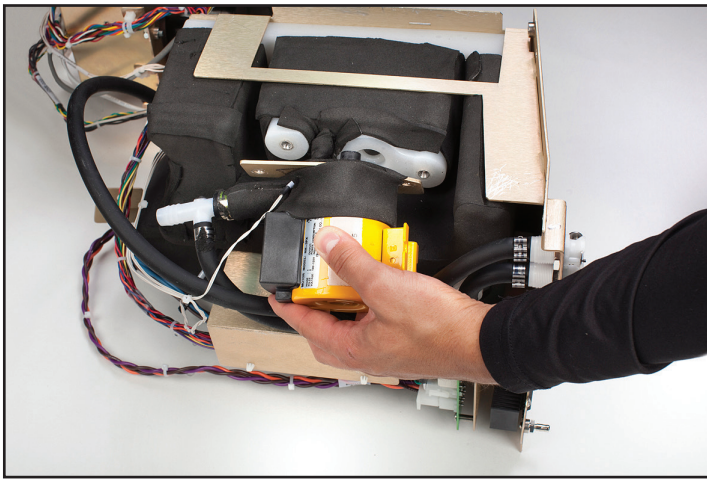
Fig. 8-42 Retirada de la bomba de refrigeración
