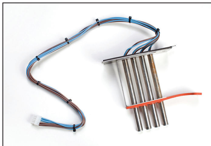
Fig. 8-48 Calentador
