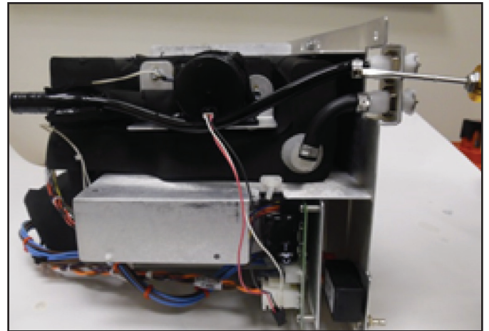
Fig. 8-45 Afloje la abrazadera (paso 3)
