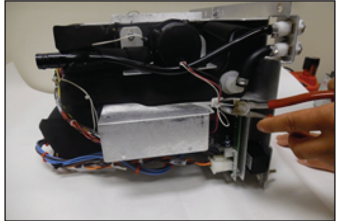
Fig. 8-44 Corte la brida de los cable (paso 2)
