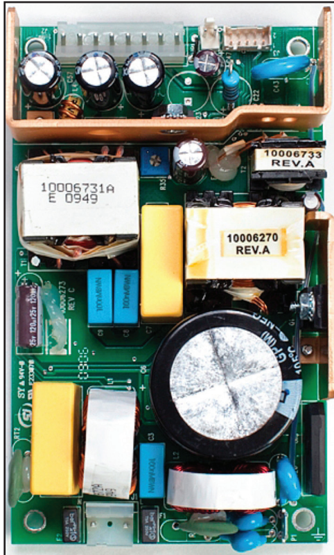
Abb. 8-66 Spannungsversorgungsmodul
