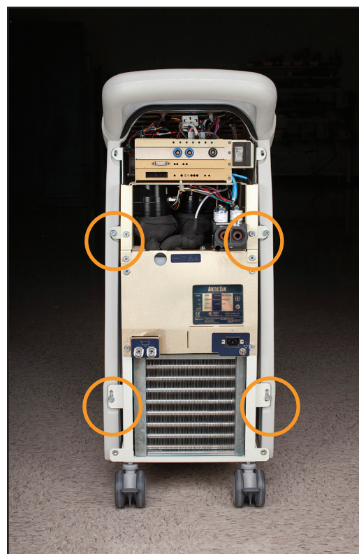
Abb. 8-11 Entfernung von 4 Schrauben (Schritt 1)
