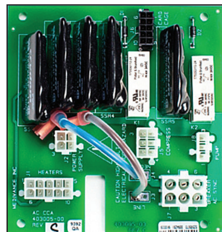
Abb. 8-7 Netzspannungsleiterplatte
