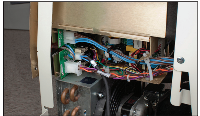
Abb. 8-20 Abtrennen des grauen Kabels des Kühler-Stromanschlusses; Position angegeben (Schritt 2)
