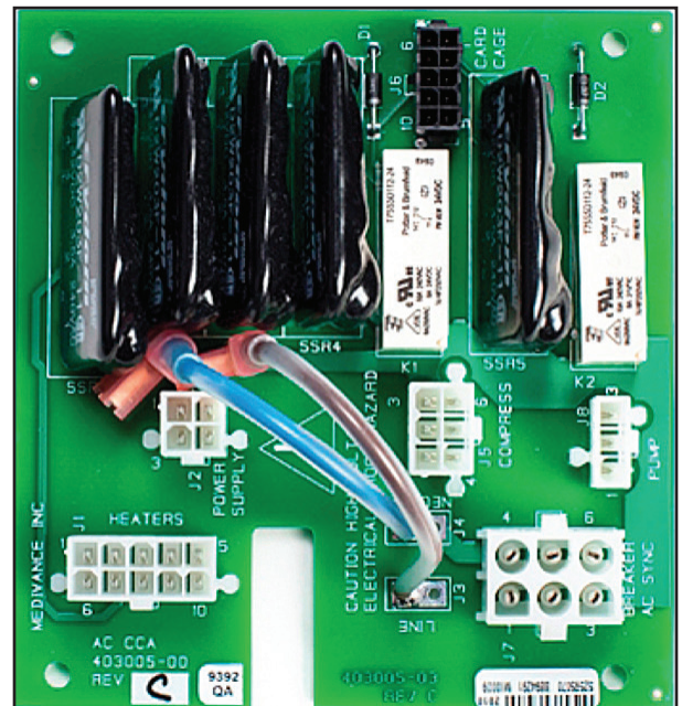
Abb. 8-68 Netzspannungsleiterplatte
