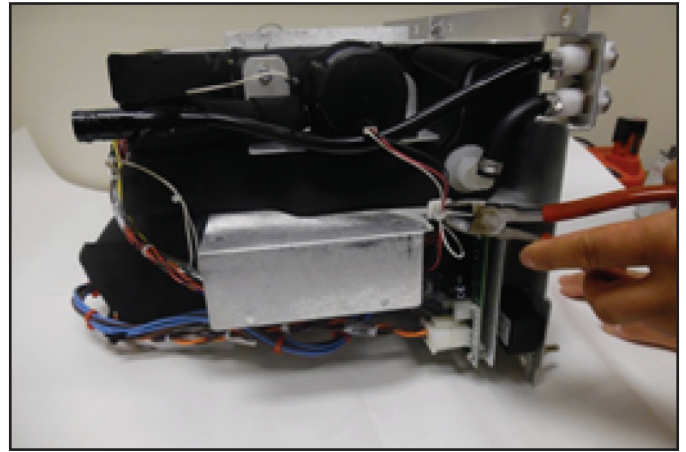
Abb. 8-44 Durchtrennen der Kabelbinder (Schritt 2)
