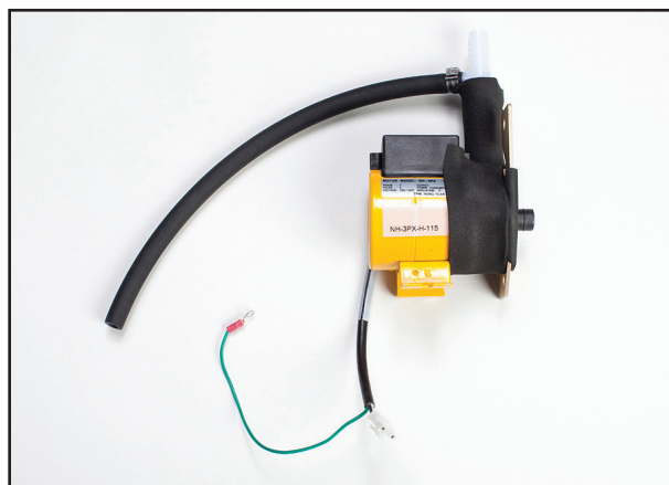
Abb. 8-39 Kühlerpumpe
