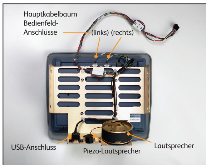
Abb. 8-55 Bedienfeld (Rückansicht)
