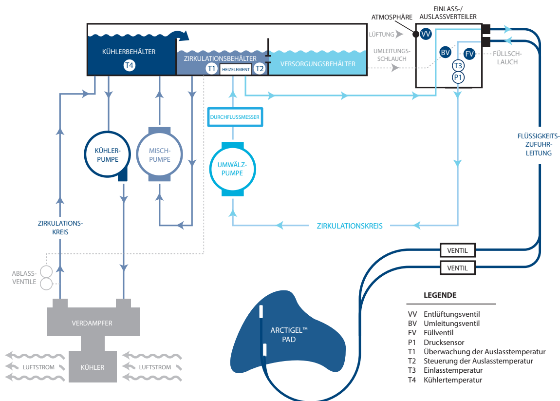
Abb. 2-1 Hydraulisches Schema
