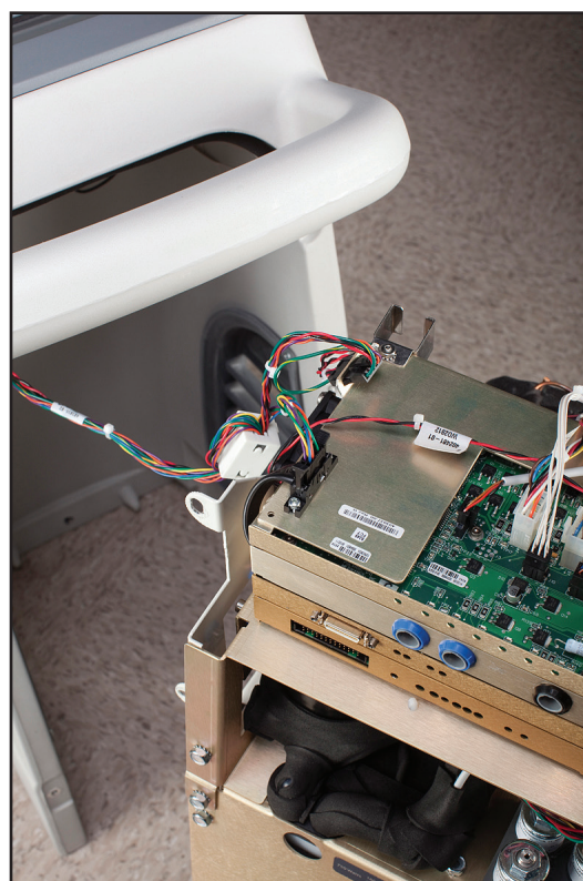
Abb. 8-12 Zu entfernende Kabelbäume (Schritt 3)
