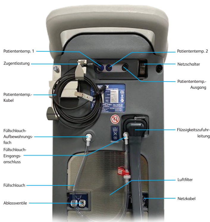
Abb. 1-1 Steuerungsmodul des ARCTIC SUN™ Temperaturmanagementsystems
